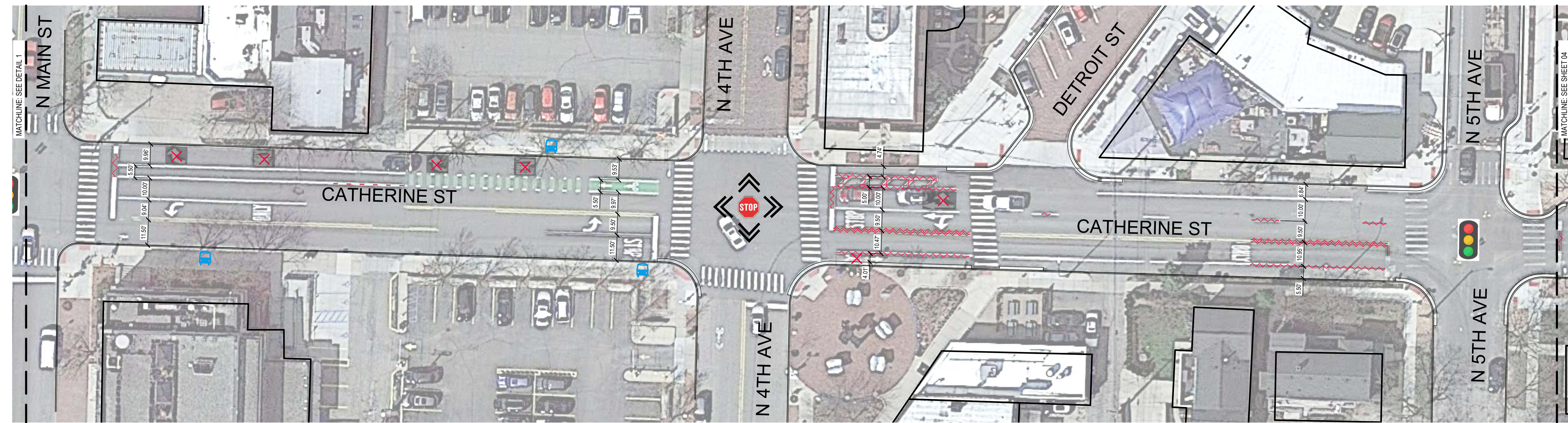
2 EXISTING MILLER - CATHERINE 2 SCALE: 1" = 20'
