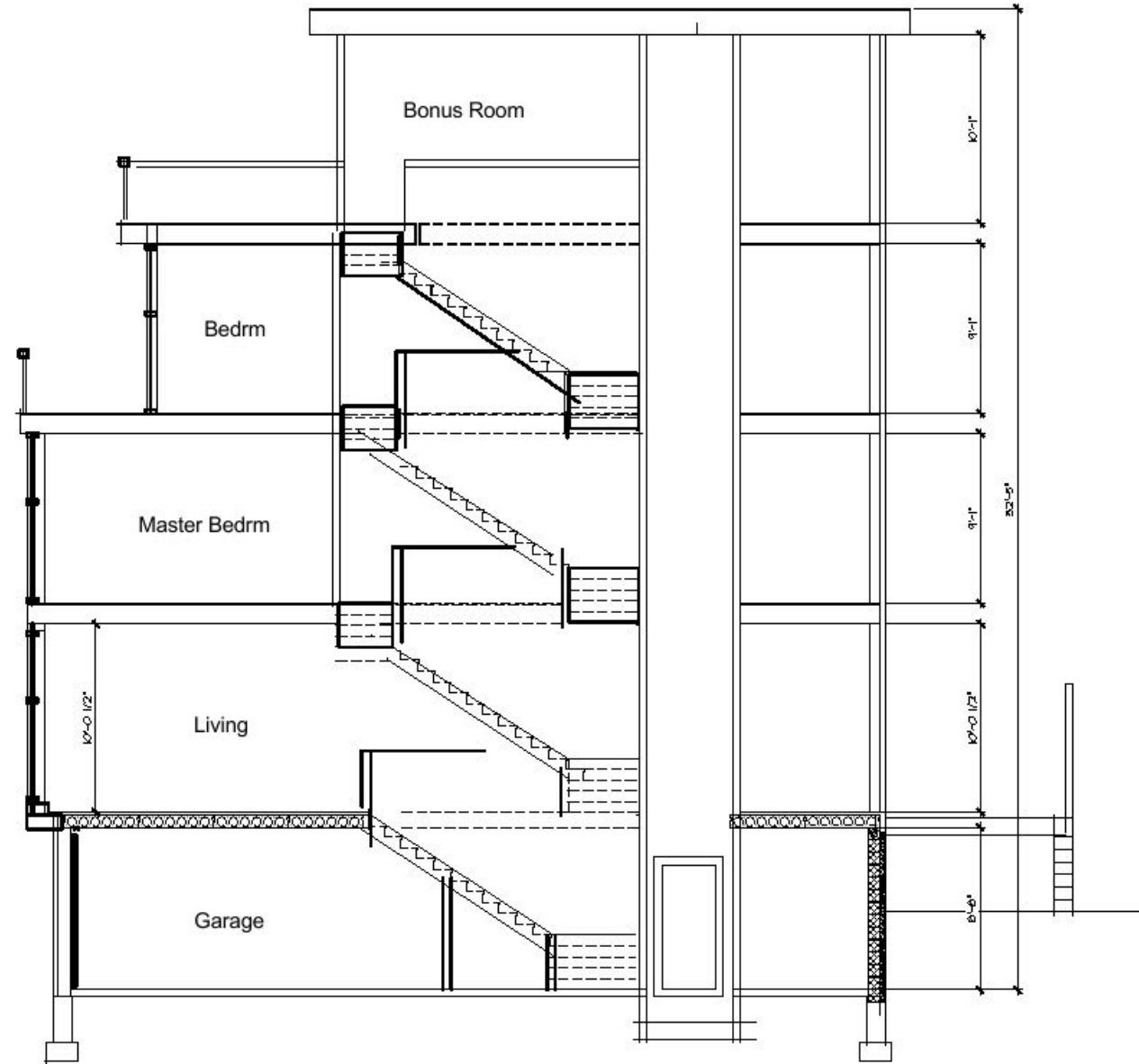
SECTION SCALE: 1/4" = 1' - 0"
