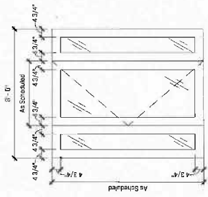
Door Type D5
