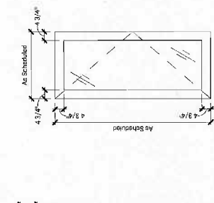
Door Type D3
